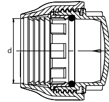
KABLİN KÖR TAPA END CAP
