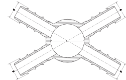
KURTAĞZI ÇOKLU DAĞITIM NİPELİ BARBED MULTICOUPLING NIPPLE
