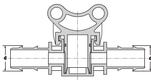
MİNİ VANA KURTAĞZI MINI VALVE BARBED
