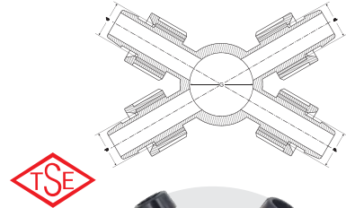
DAMLAMA ÇOKLU DAĞITIM NİPELİ DRIPLINE MULTICOUPLING NIPPLE
