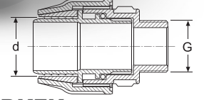
LAYFLAT ERKEK LAYFLAT MALE ADAPTOR
