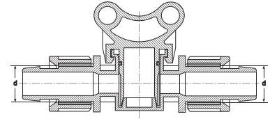
MİNİ VANA YASSI DAMLAMA MINI VALVE TAPE
