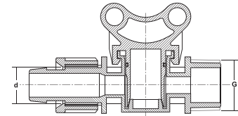
MİNİ VANA YASSI DAMLAMA - ERKEK MINI VALVE TAPE - MALE
