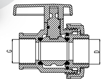
KÜRESEL VANA DIŞI - DIŞI BALL VALVE FEMALE - FEMALE
