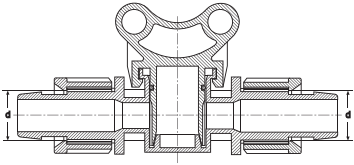
MİNİ VANA DAMLAMA MINI VALVE DRIPLINE
