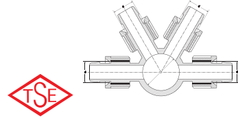
DAMLAMA ÇOKLU DAĞITIM NİPELİ DRIPLINE MULTICOUPLING NIPPLE
