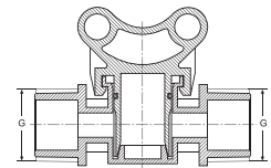
MİNİ VANA ERKEK MINI VALVE MALE
